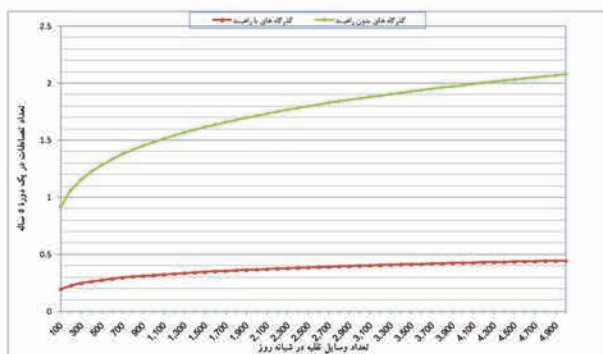
شکل ۲. روند تغییر تعداد تصادفات با تعداد وسایل نقلیه عبوری در شبانه‌روز بر اساس مدل ۲۲. (محاسبه شده با: تعداد قطارهای عبوری در شبانه‌روز = 20 ، موقعیت گذرگاه برون‌شهری، متوسط سرعت قطارها بیش از 60 \text{ km/h} ، نوع روسازی جاده = آسفالتی)
