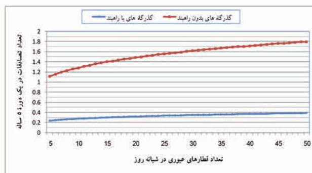
شکل ۳. روند تغییر تعداد تصادفات با تعداد وسایل نقلیه عبوری در شبانه‌روز بر اساس مدل ۲۲. (محاسبه شده با: تعداد وسایل نقلیه عبوری در شبانه‌روز = 1000 ، موقعیت گذرگاه برون‌شهری، متوسط سرعت قطارها بیش از 60 \text{ km/h} ، نوع روسازی جاده = آسفالتی)
