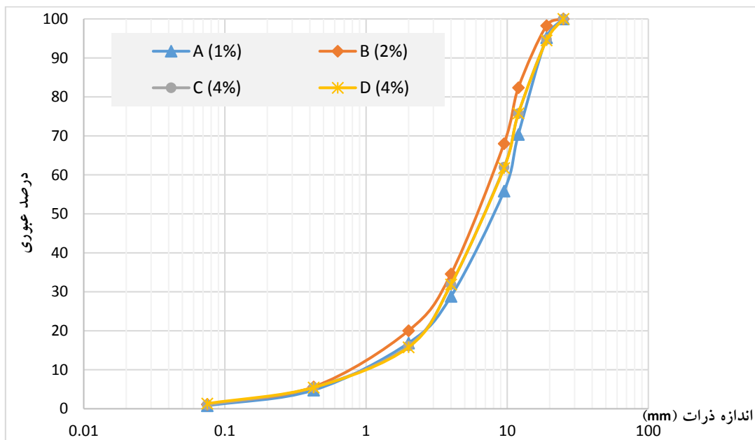
شکل ۴. دانه‌بندی اولیه مصالح بازیافتی
