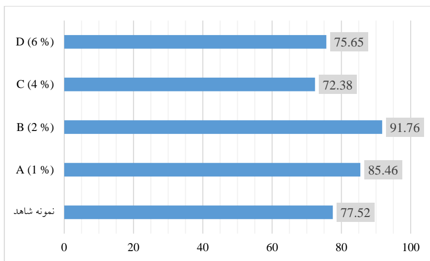
شکل ۷. نتایج CBR آزمایشگاهی مصالح (درصد)
