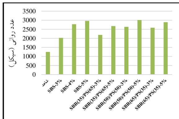
شکل ۱۳. نتایج آزمون خزش دینامیکی
