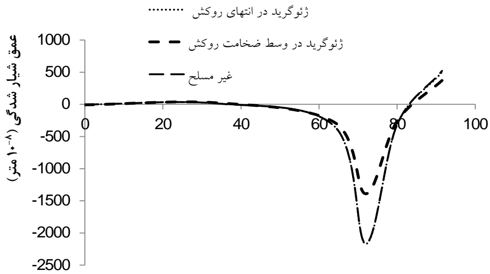
شکل ۱۰. تاثیر ژئوگرید بر پروفیل تغییر شکل سطح روکش
