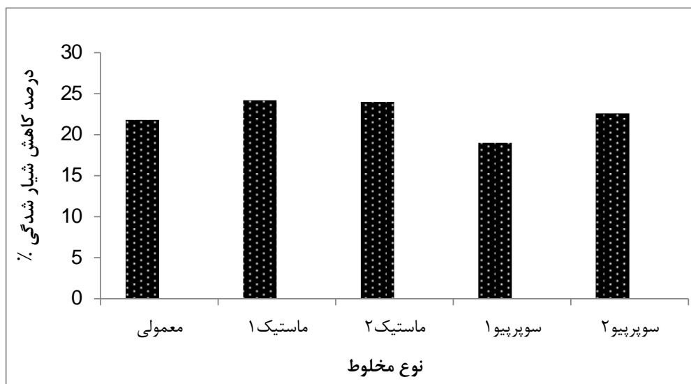
شکل ۱۳. درصد کاهش شیار شیب در روکش به ضخامت ۶ سانتیمتر که ژئوگرید در وسط لایه قرار گرفته است
