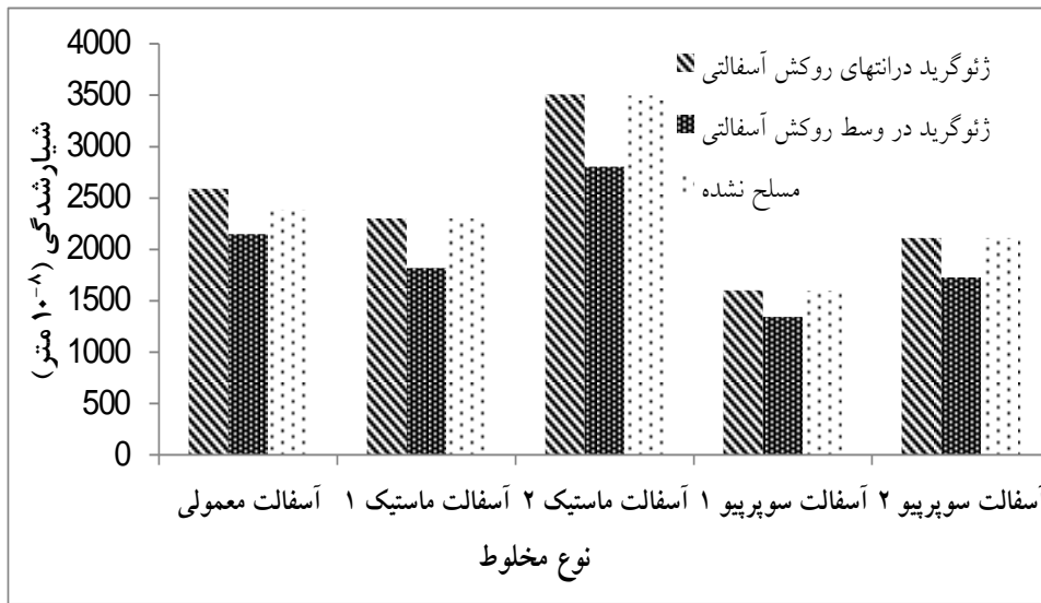
شکل ۱۲. تاثیر ژئوگرید بر عمق شیار شیب بر مخلوطهای مختلف
