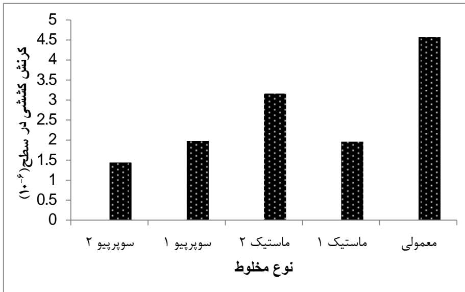
شکل ۷. حداکثر گرنش کشتی در سطح برای مخلوطهای مختلف
