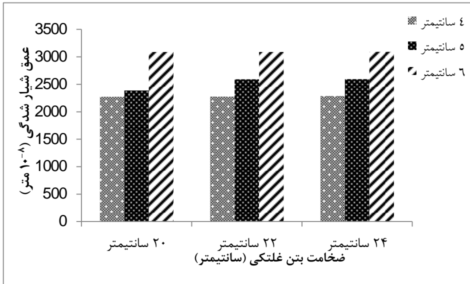
شکل ۱۶. تاثیر ضخامت روکش و لایه بتن غلتکی بر عمق شیاردگی حداکثر
