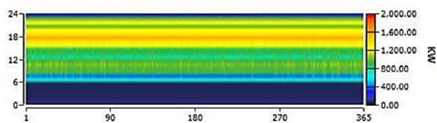
شکل ۱۶. انرژی خریداری شده از شبکه در طول سال در سیستم پیشنهادی
