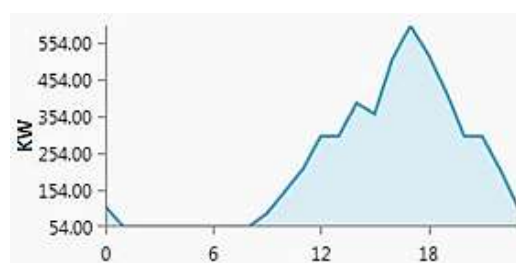
شکل ۹. بار مصرفی ایستگاه شارژ سریع DC خودرو الکتریکی
