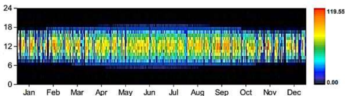
شکل ۱۱. توان خروجی PV در طول سال در سیستم پیشنهادی
