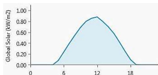
شکل ۱۲. تابش خورشید در طول یک روز نمونه در سیستم
