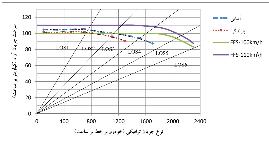
شکل ۶. منحنی میانگین سرعت جریان آزاد-نرخ جریان در دو وضعیت آب‌وهوای بارانی و آفتابی
