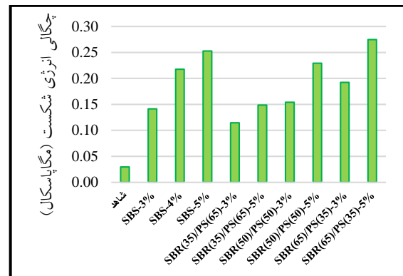
شکل ۱۲. چگالی انرژی شکست نمونه‌های آسفالتی
