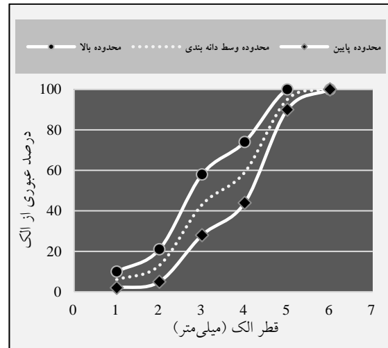
شکل ۱. حدود بالا، پایین و وسط دانه‌بندی شماره ۴ نشریه ۲۳۴
